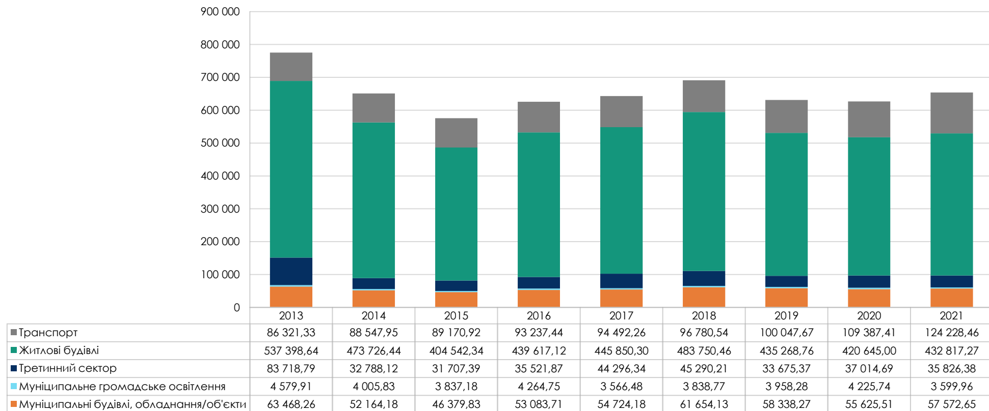
Рис. 3.10. Динаміка викидів CO 2 у 2013-2021 роках в обраних секторах, TCO 2
