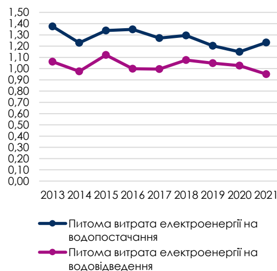
Рис. 2.16. Питомі витрати електроенергії на водопостачання та водовідведення, кВт*год/м 3
