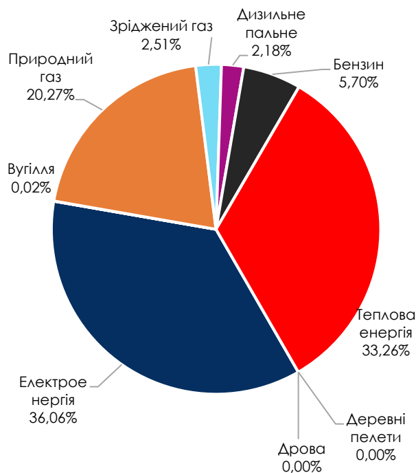
Рис. 3.9. Розподіл викидів CO 2 залежно від енергоресурсу у базовому 2013 році
