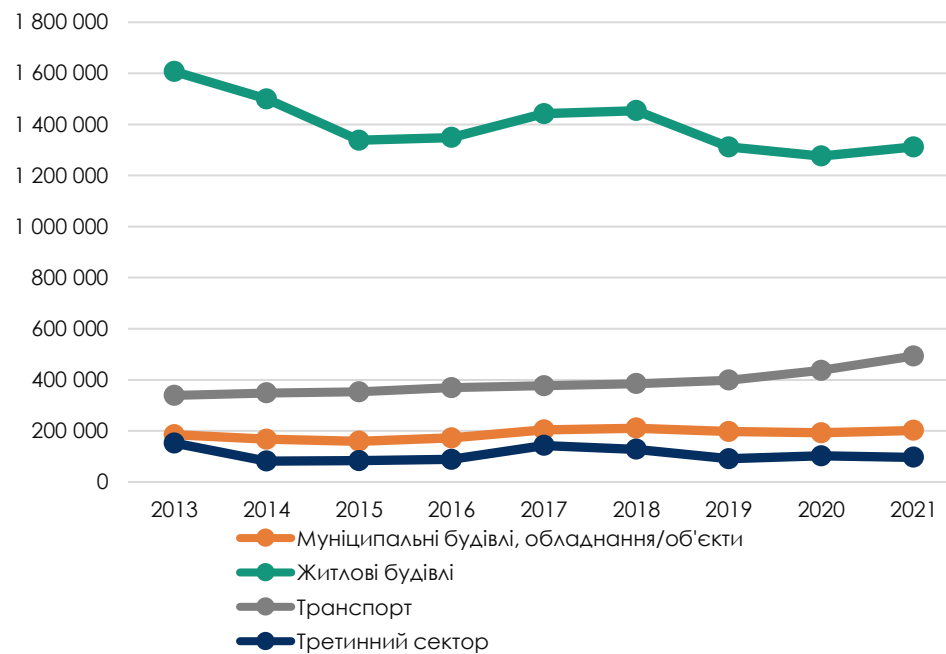
Рис. 3.7. Динаміка споживання енергоресурсів за 2013-2021 роки, МВт*год
