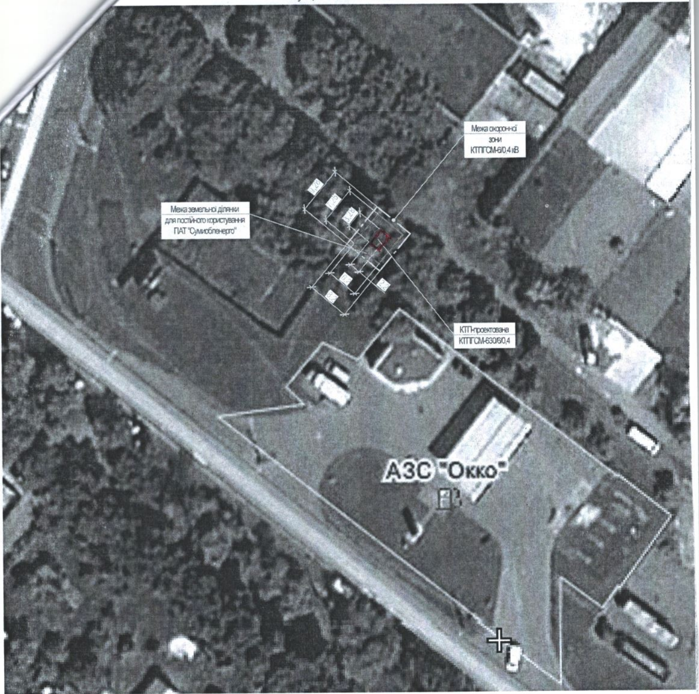
Відомість відводу землі під проектовану КТПГСМ-6/0,4 кВ
